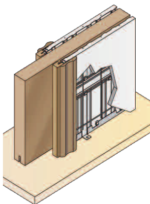
CONTROTELAI PORTE SCORREVOLI INTERNO MURO MOD. NEW SPACE DIERRE PRONTI A MAGAZZINO
